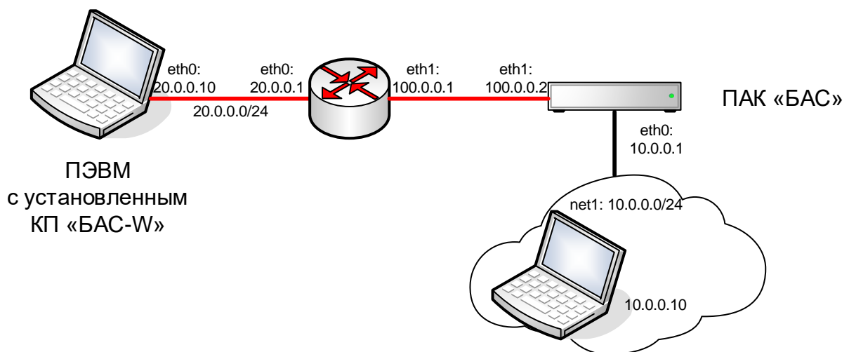
Рисунок 1 – Схема стенда
