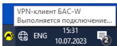
Рисунок 14 – Подключение VPN-профиля
