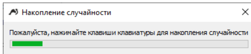
Рисунок 6 – Накопление случайности
