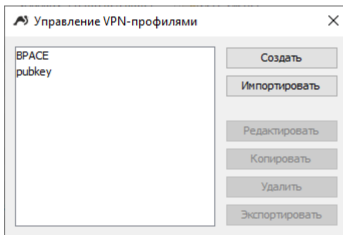
Рисунок 8 – Управление VPN-профилями
