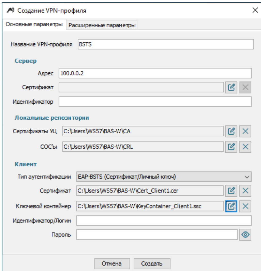
Рисунок 10 – Настроенный VPN-профиль
